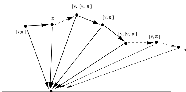
FIG. 39 – Graphe de type Bernoulli non fermé
