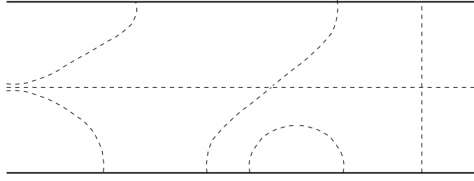
FIG. 40 – Géodésiques dans la bande
