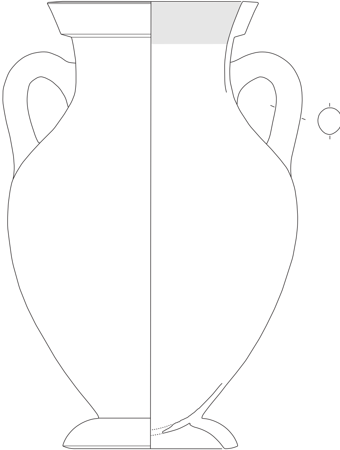
173 | Profilzeichnung der Amphora B Kat. 13 mit eingesetztem, möglicherweise zugehörigem Mündungsfragment, Massstab 1:3.
