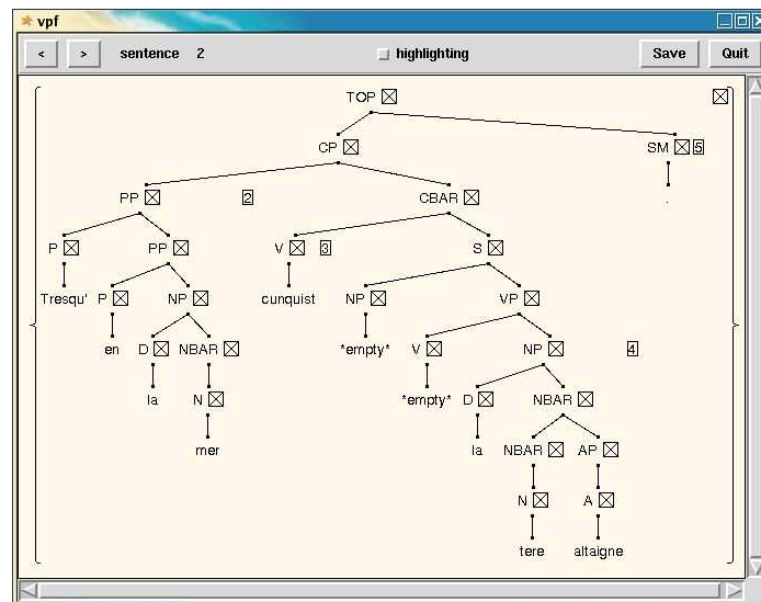
Fig. 2. YAP parser output
