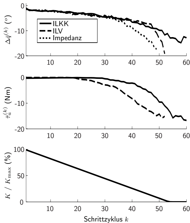
Bild 5 Vergleich der mittleren Winkelabweichung \Delta \bar{q} während der Standphase im rechten Kniegelenk (oberes Diagramm) sowie der mittleren adaptierten Unterstützung \bar{\tau}_u^{(k)} (mittleres Diagramm) unter den drei Konditionen IMPEDANZ, ILV und ILKK. Das untere Diagramm zeigt die während des Experiments unter allen Konditionen linear reduzierte Steifigkeit des Impedanzreglers als Prozentsatz der maximalen Steifigkeit K_{max} .
