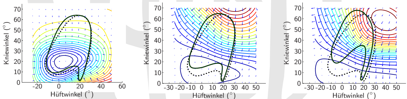
Bild 6 Projektionen des ILKK auf den zweidimensionalen Raum für das rechte Bein nach Schrittzklus k = 20 (links), 40 (Mitte) und 60 (rechts). Für die Projektionen werden die Koordinaten des linken Beins auf 15^\circ Hüftflexion und 62^\circ Knieflexion (Mitte Schwungphase) festgehalten, während für die Koordinaten des rechten Beins beliebige Winkel zugelassen werden. Die Pfeile illustrieren die auf Hüft- und Kniegelenk des rechten Beins bezogenen Komponenten des negativen Gradienten des durch Höhenlinien angedeuteten Potentials. Die gestrichelte, schwarze Linie markiert den Verlauf der Referenztrajektorie, während die durchgezogene, schwarze Linie den Verlauf der Ist-Winkel für den entsprechenden Schrittzklus wiedergibt.
